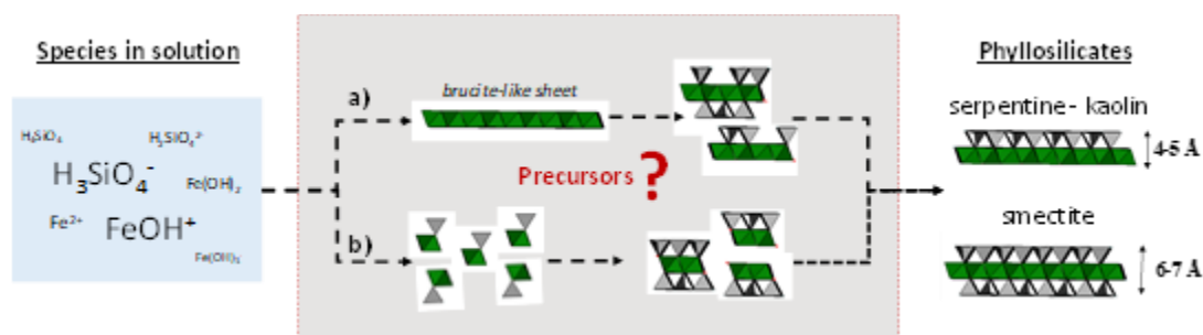
Figure 1 : Représentation schématique des possibles chemins de formation des phyllosilicates ferreux à pH basique.
